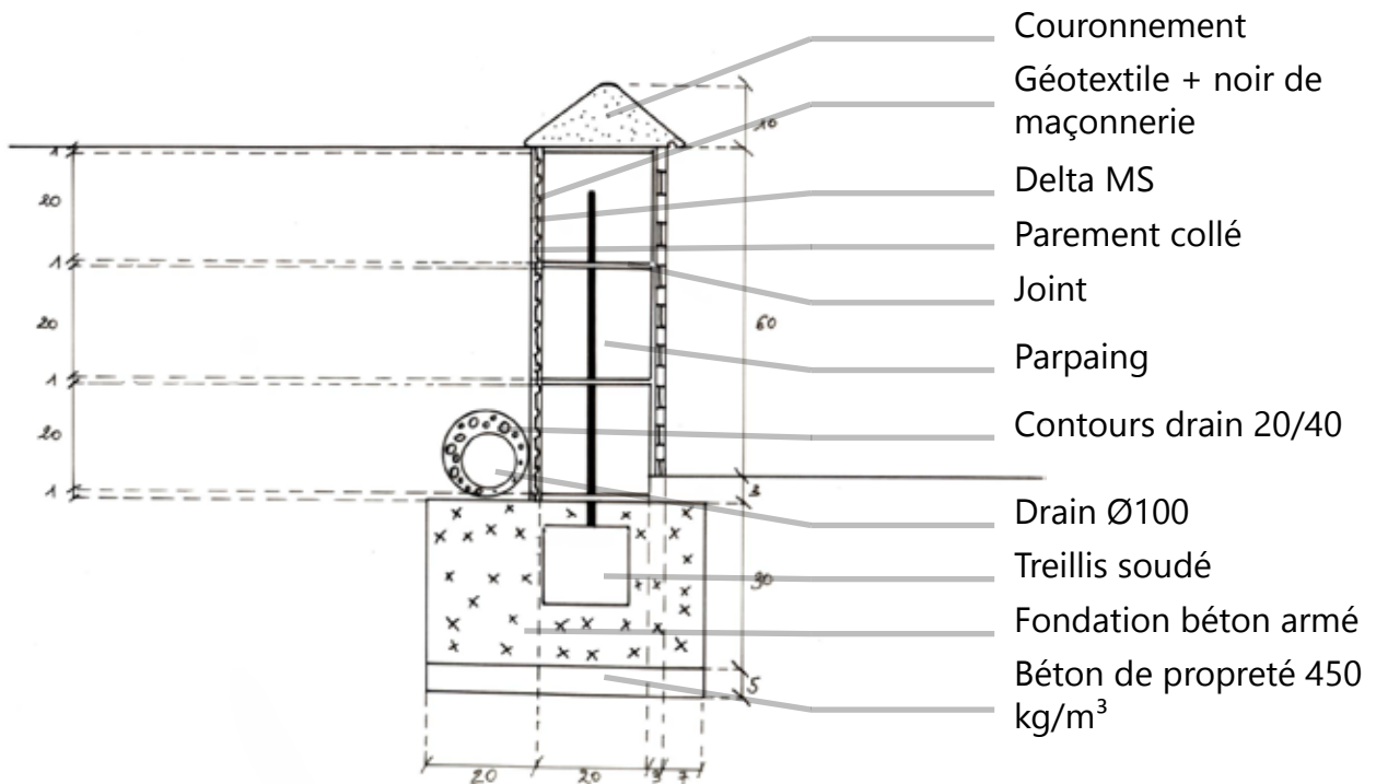
Coupe technique d'un muret. Projet non réalisé
