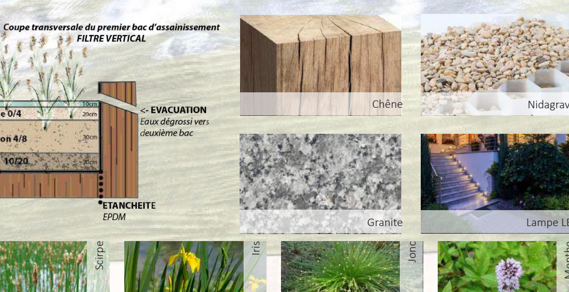
Coupe transversale du premier bac d'assainissement
