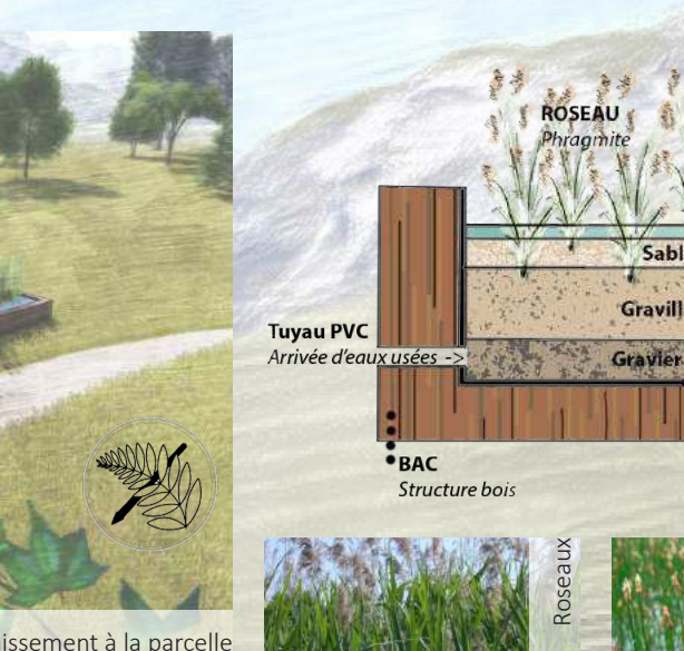
Coupe transversale du premier bac d'assainissement
