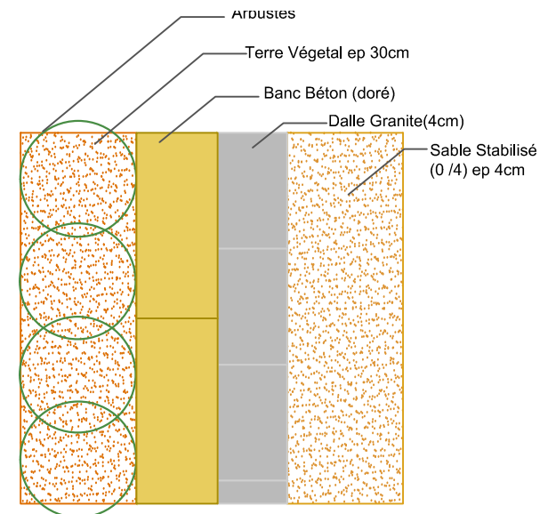
Vue du haut 1/20
