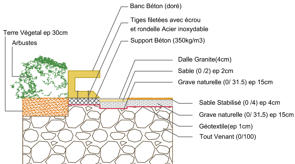
Diposition Banc Béton 1/50
