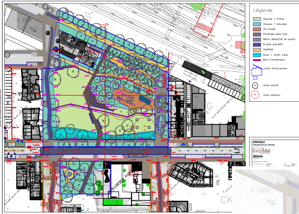
Plan masse du parc Grenoble Cambridge. A0/200e
