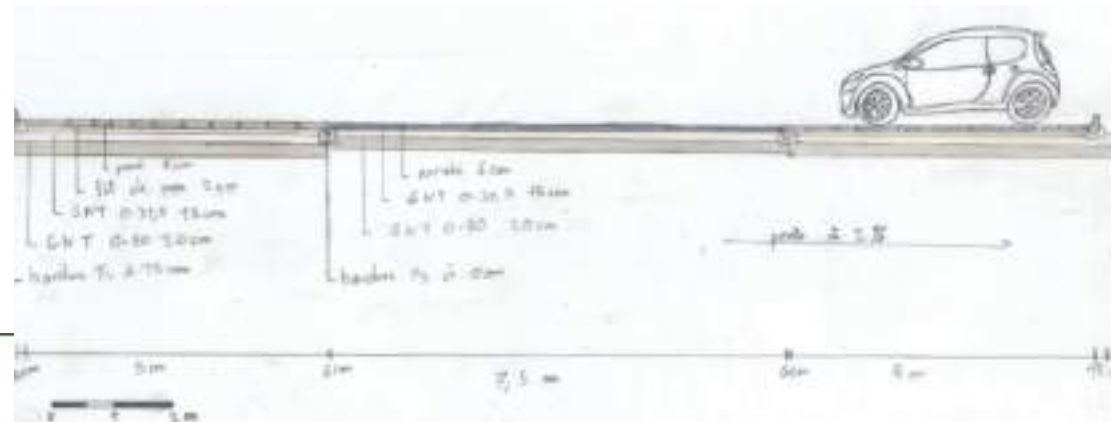
Coupe technique du parking 1/50
