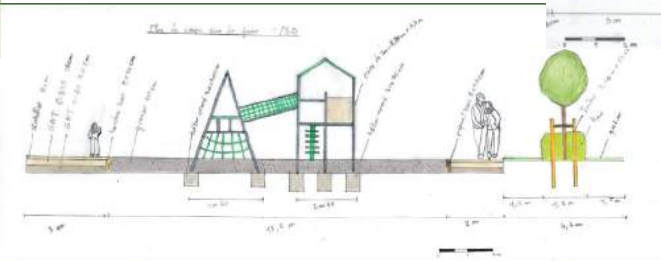
Coupe technique de l'aire de jeu 1/50
